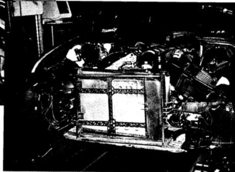
Auch wenn es für manchen eher wie eine Unfallinstandsetzung aussieht, sind das doch die notwendigen Demontagearbeiten zur Nachrüstung einer Klimaanlage.
