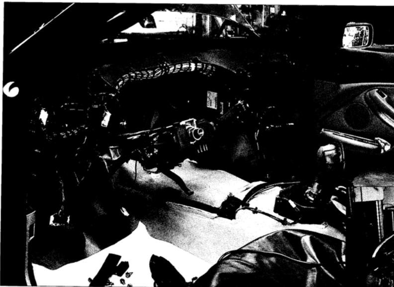
Um das Lüftungssystem ausbauen zu können, entfernen die Weileder-Mechaniker bei diesem 5er-BMW die Mittelkonsole und das komplette Armaturenbrett.
